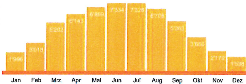
Jährliche Stromproduktion (kWh)
